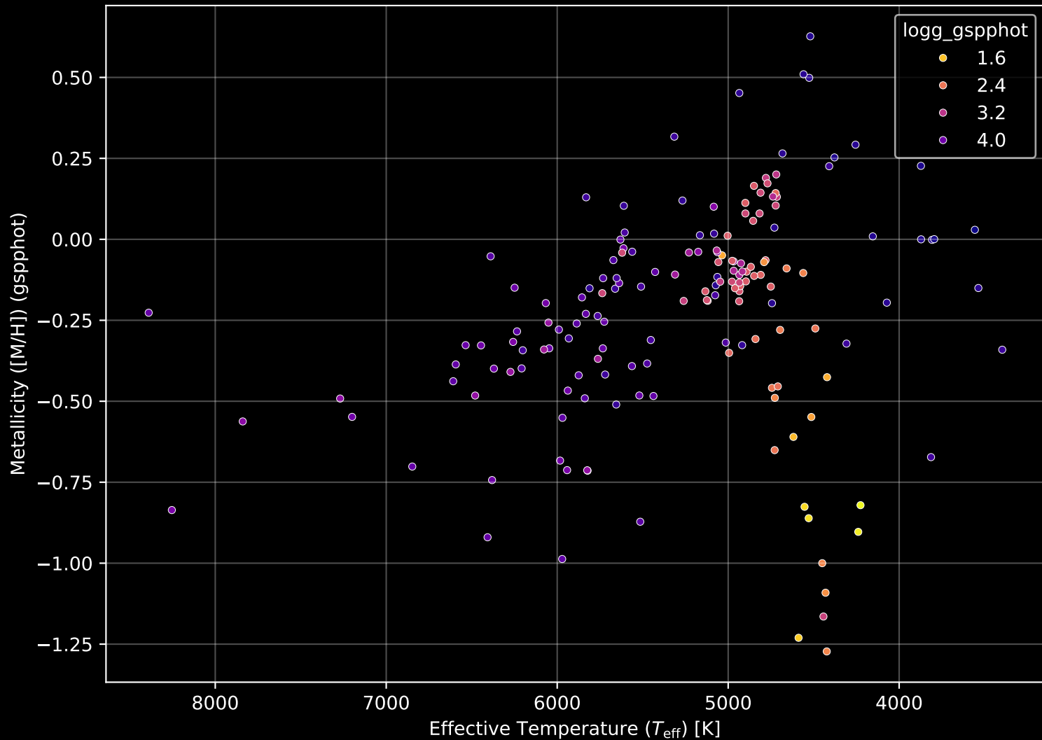
APOGEE DR17 Field: [286-25-O_TESS] Stellar Population Parameters (n= 166)
