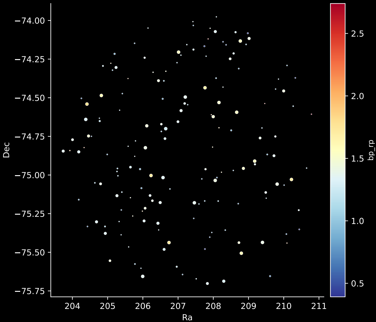
APOGEE DR17 Field: [286-25-O_TESS] Stars: 166
